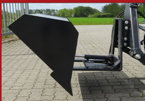
Frontskovlen tømmes let, ved hjælp af en stærk centermonterede hydrauliske cylinder.
