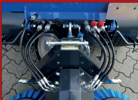
Fejesusgefronten er opbygget med standard A-ramme og kan leveres med 2, 3 eller 4 børster.
