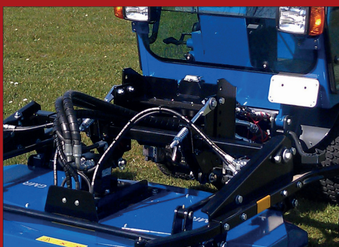
Som tilvalg kan klippehøjden indstilles hydraulisk og betjenes let og enkelt af chaufføren, direkte fra kabinen
